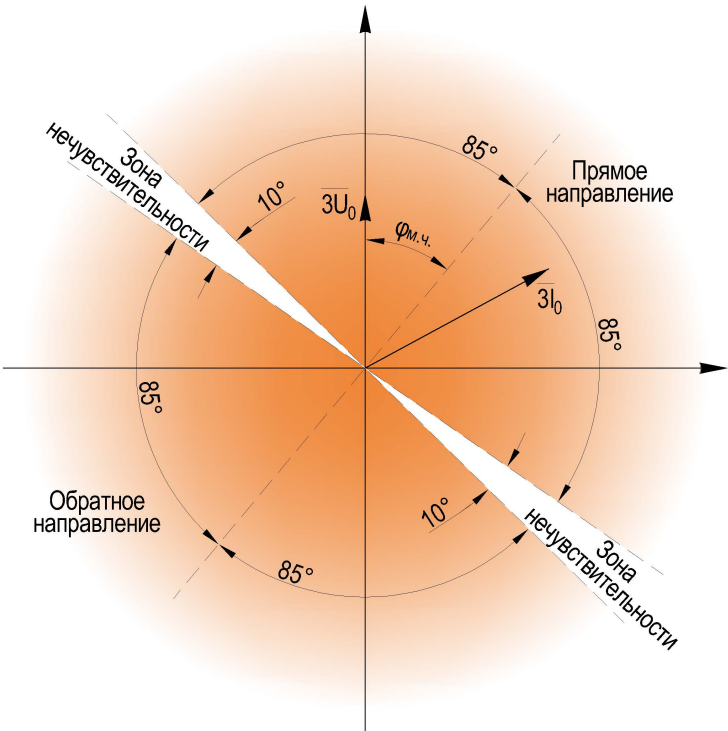
Рисунок 2.30 – Характеристика органа направления мощности нулевой последовательности 2.11.3.8 Алгоритм работы функции «ОНМ НП» выполнен в соответствии с рисунком 2.31. В таблице 2.24 приведены параметры, необходимые для настройки функции «ОНМ НП».
